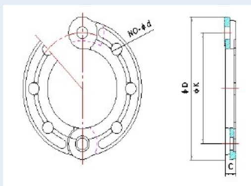
BRIDA LATERAL SECCIONADA/LOOSING FLANGE
